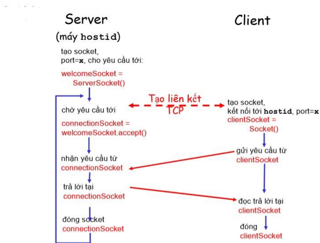
Hình 2: Hoạt động của TCP Socket trong mô hình client-server
